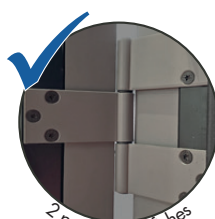
2 paumelles 3 fiches
